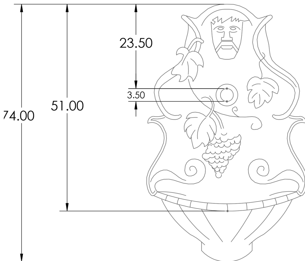
Elülső nézet
